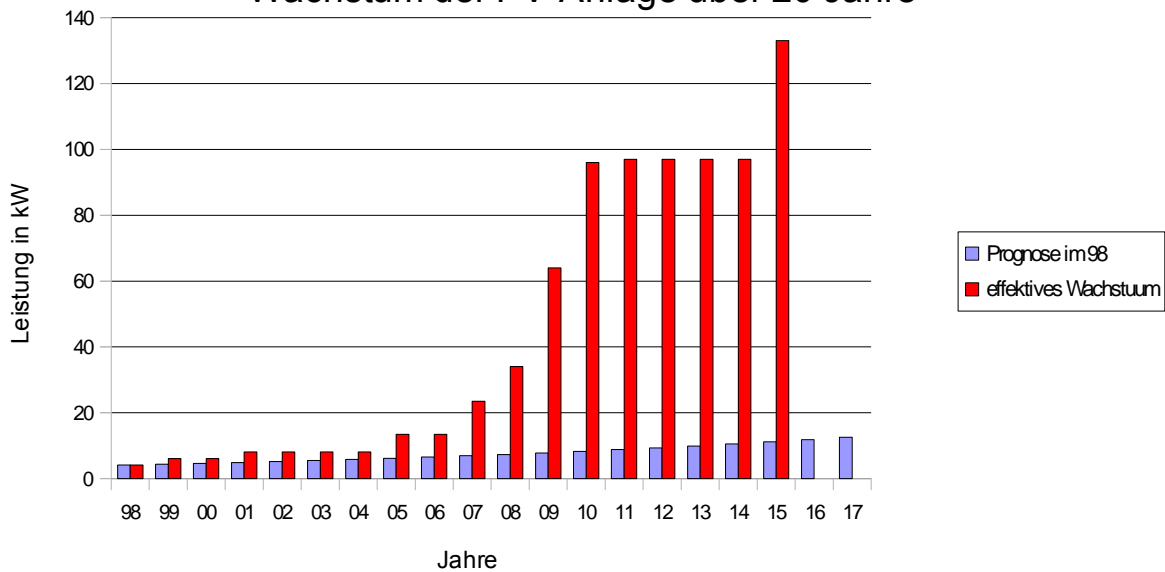
Wachstum der PV-Anlage über 20 Jahre
