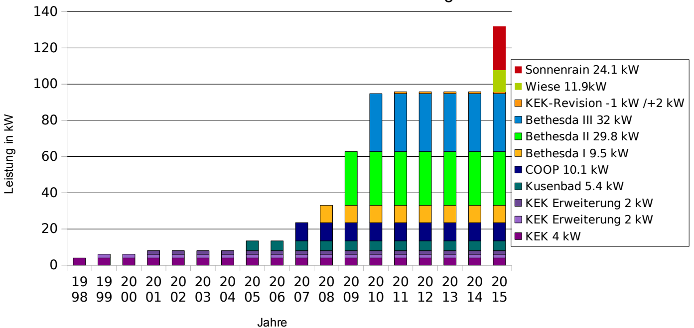
Zuwachs der einzelnen PV-Anlagen
